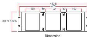
LSA+ Rack Mount Back Mount Frame เป็นที่ติดตั้งไว้กับตู้ Rack 19" มาตรฐานทั่วไป ใช้สำหรับติดตั้งอุปกรณ์ระบบโทรศัพท์เข้ากับระบบคอมพิวเตอร์ไว้ในตู้เดียวกันกับระบบเครือข่ายคอมพิวเตอร์
