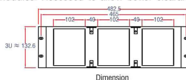
LSA+ Rack Mount Back Mount Frame ชุดที่ติดตั้งได้กับตู้ Rack 19" มาตรฐานทั่วไป ใช้สำหรับติดตั้งแผงระบบโทรศัพท์และระบบคอมพิวเตอร์ไว้ในตู้โดยกับระบบเครื่องข่ายคอมพิวเตอร์
